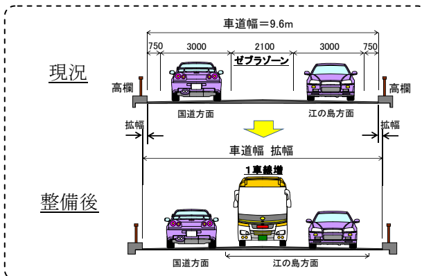
<江の島大橋改修工事の概要>
